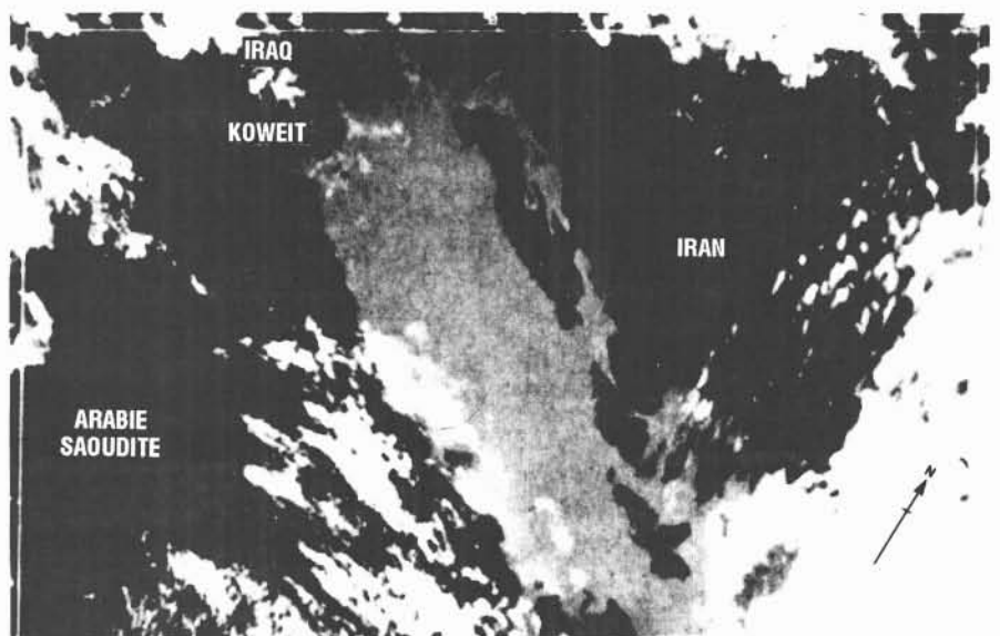
Prise en juin 1983, cette photo satellite montre la dispersion du pétrole à la suite d'un écoulement désastreux survenu dans le champ pétrolier Nowruz, au nord-est du golfe. Les accidents plus récents ont pour leur part eu lieu dans le nord-ouest.
